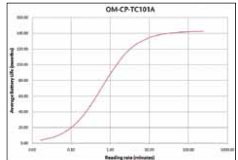
Vida útil promedio de la batería frente velocidad de lectura del OM-CP-TC101A registrando en un entorno de 25 °C.
